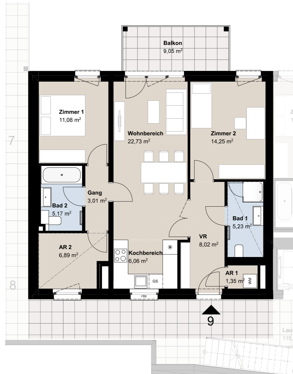
1. Obergeschoss
